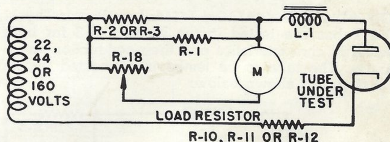
Fig. 3—Diode & Rectifier Test Circuit
